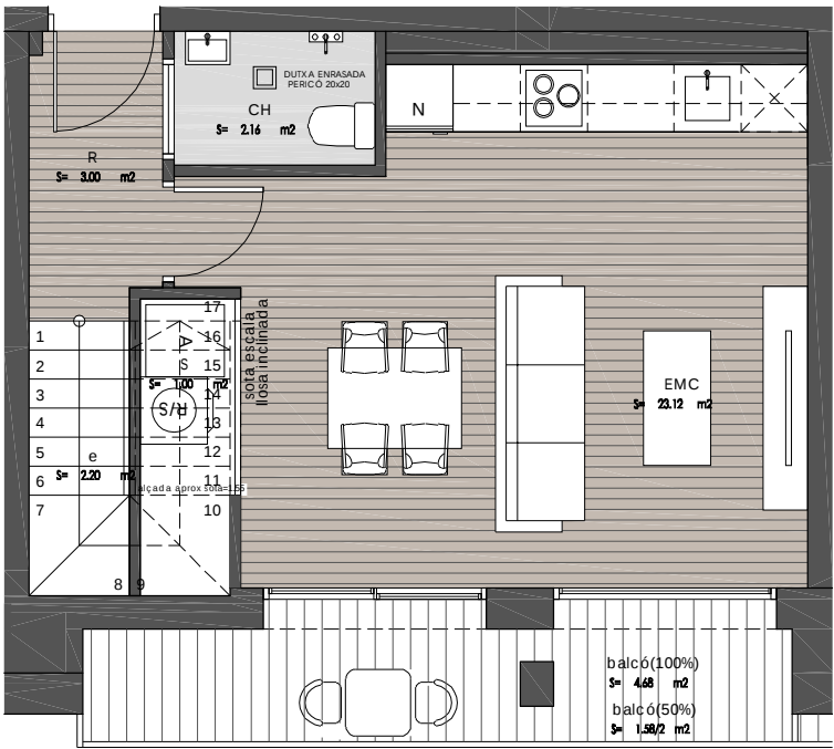
PLANTA TERCERA C/ DE TARRAGONA
