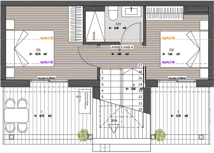
PLANTA SOTACOBERTA C/ DE TARRAGONA
