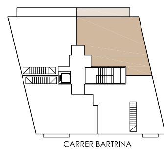
PLANTA TERCERA PATI INTERIOR D'ILLA
